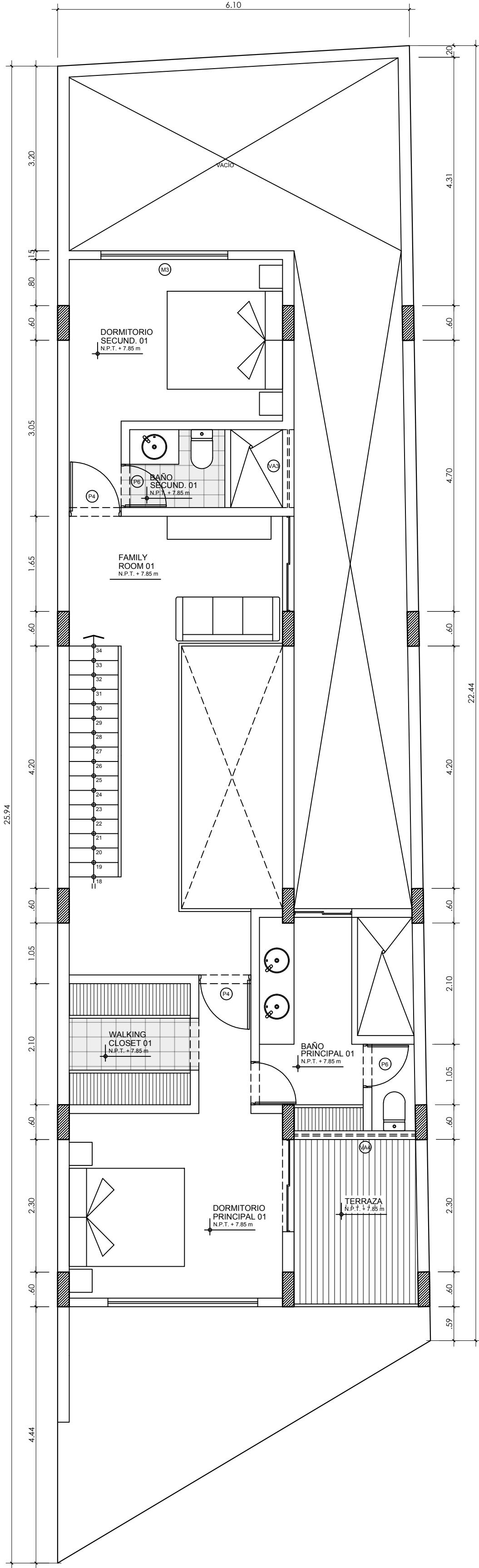
AREA TECHADA: 90.89 M2 TERCER NIVEL N.P.T. + 07.85 m
